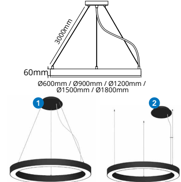
Bijgeleverde pendelset kan zowel als optie 1 en 2 worden gemonteerd
