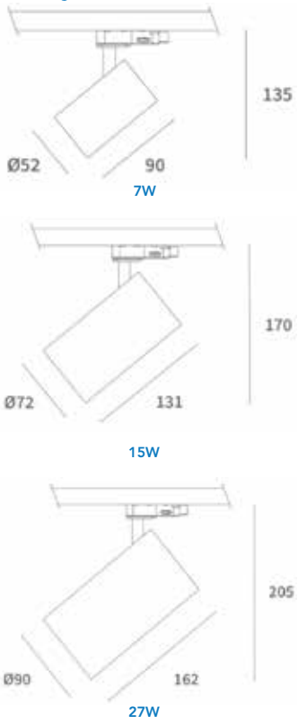
Maattekening:
