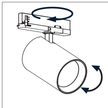
355° draaibaar / 90° zwenkbaar
